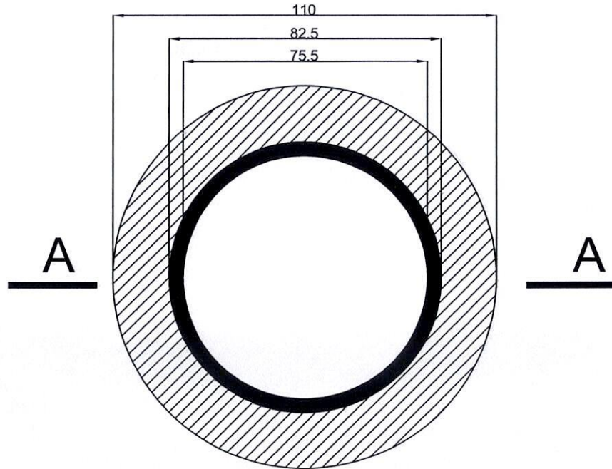
MẶT BẰNG
