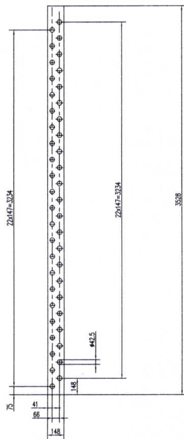
Chi tiết Tấm liên kết ống
