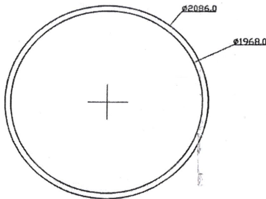
Vành tăng cứng 1 - số lượng 1 cái Khối lượng 24kg Vành tăng cứng hình tròn Thép 310S, dày 8 mm
