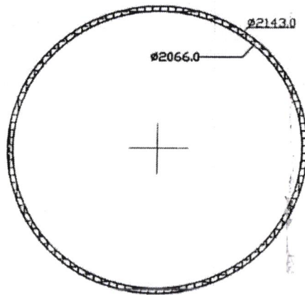
Vành tăng cứng 1 - số lượng 1 cái Khối lượng 17kg Vành tăng cứng hình tròn Thép 310S, dày 8mm
