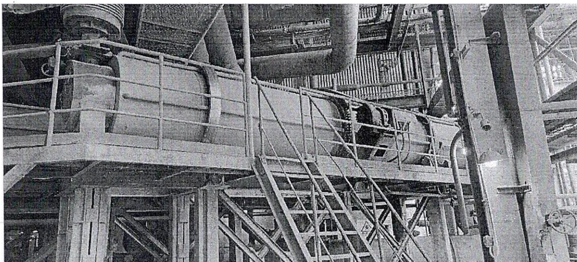
Hình ảnh bộ làm mát xỉ đáy lò (lò hơi số 4)
