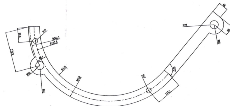
GIÁ ĐỠ SÀN NGHIÊN B vật liệu đúc giá đỡ là thép C85
