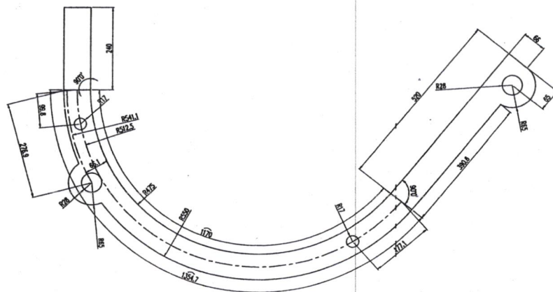
GIÁ ĐỠ SÀN NGHIÊN A vật liệu đúc giá đỡ là thép C85
