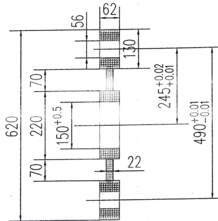
MC A-A
