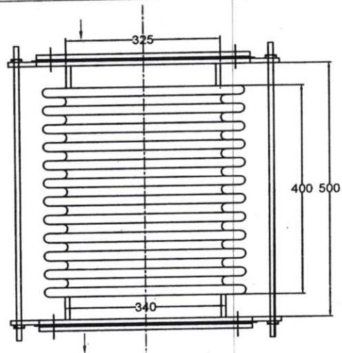
KHỚP GIẢN NỖ ỚNG CẤP THAN VÀO LÒ
