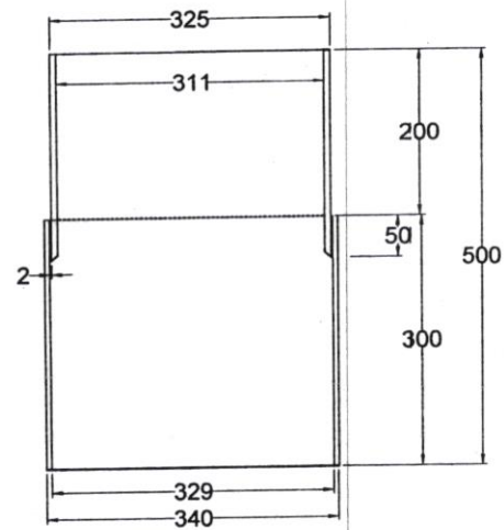
CHI TIẾT ỚNG LÒNG BÊN TRONG KHỚP GIẢN NỖ
