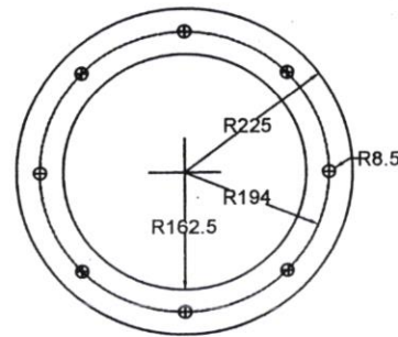
BÍCH ĐẦU VÀO
