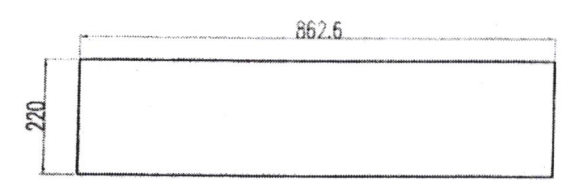
Tay giữ cánh van loại 1 Vật liệu SUS 304, thép dày 18mm
