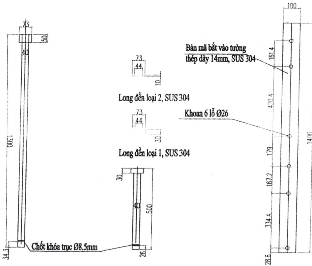
Trục loại 1 Vật liệu SUS 304
