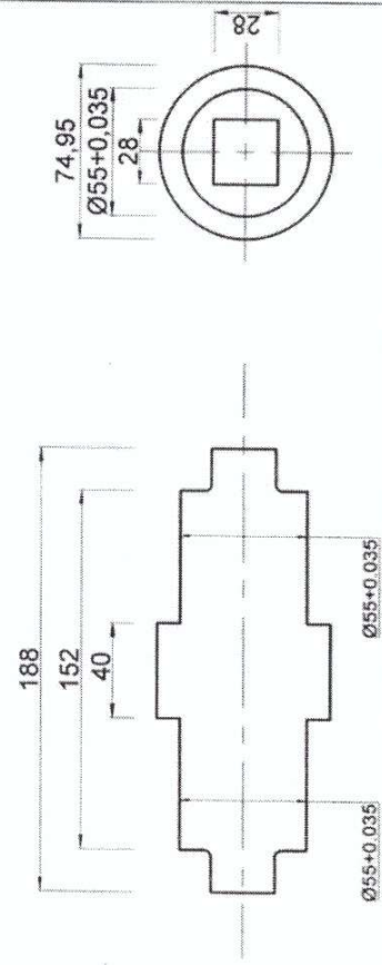
MẶT BÍCH 2 BÊN VẬT LIỆU CHẾ TẠO THÉP C45
